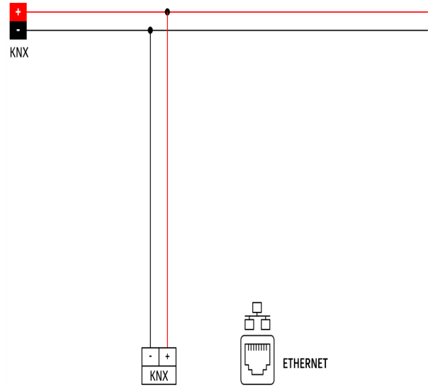
Ledningsdiagram
