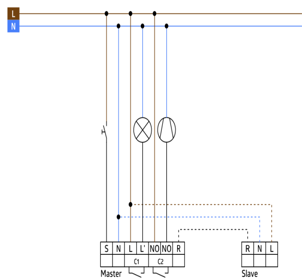
Ledningsdiagram
