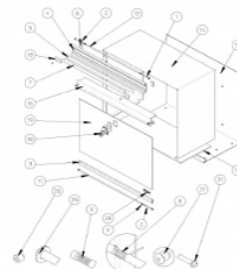
Løsdeler oversigt
