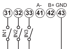
Fig. 27 Digital inputs
