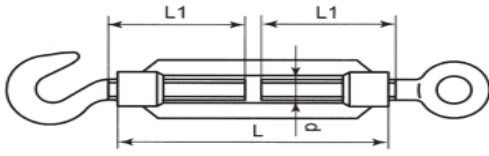
Galv. Bardunstrammer Øje/Krog, DIN 1480 Galv. Turnbuckle Eye/Hook, DIN 1480
