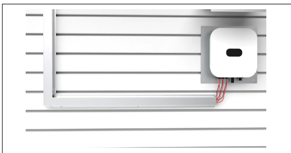
9. Placer enhver ny NM Cable Protection og tilpasse længden til ledningslængden.
